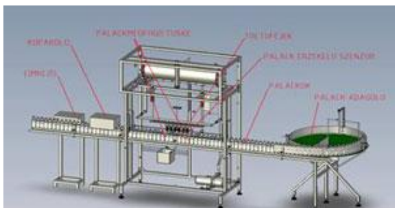
SCH-APK/... automata palackozó gép működési vázlata
